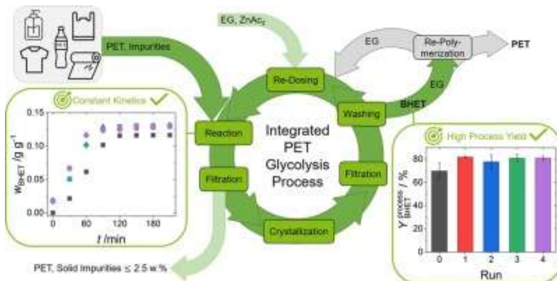
Figura 26: Esquema conceptual del proceso integrado de glicólisis catalítica de PET en circuito cerrado: reacción → filtración → cristalización → filtración → lavado → redosificación.
