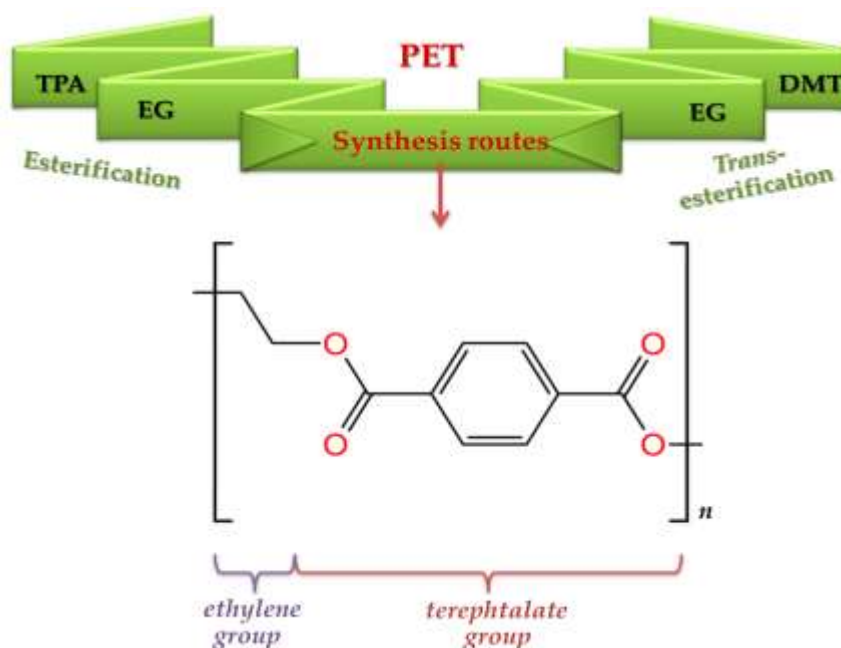
Figura 1: Rutas de síntesis del PET por esterificación directa del TPA con EG y por transesterificación del DMT con EG seguida de policondensación. Fuente: Enache y otros (2024) [1]
