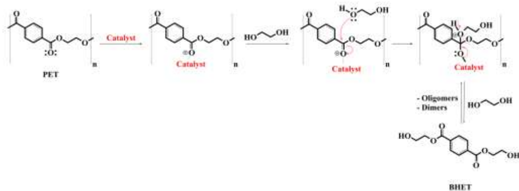
Figura 12: Mecanismo posible de la glicólisis del PET Fuente: Enache y otros (2024) [1]
