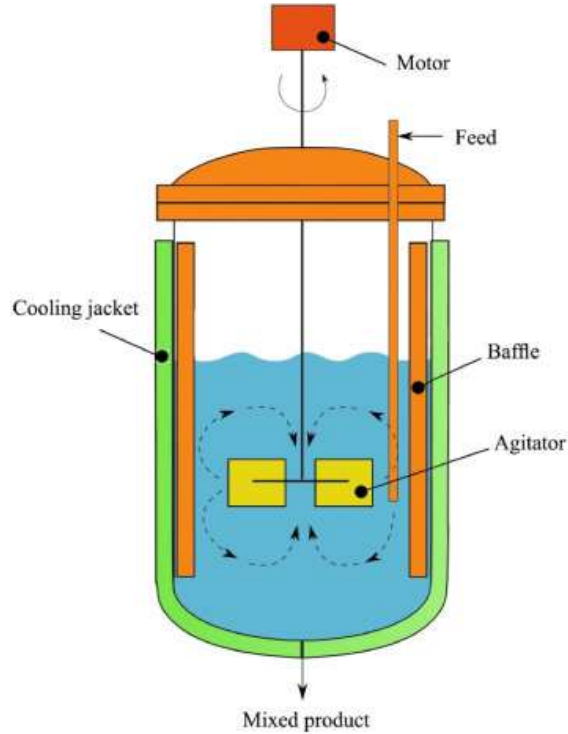
Figura 24: Configuración general de un reactor agitado encamisado batch como el seleccionado para la planta de 1 000 kg/año de BHET. Adaptado de Tabatabaei y otros (2019) [50].
