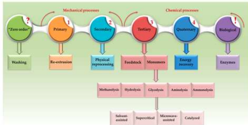
Figura 2: Diferentes métodos de reciclaje del PET basados en procesos mecánicos o químicos, con indicación de los productos finales obtenidos en cada ruta. Fuente: Enache y otros (2020) [1]
