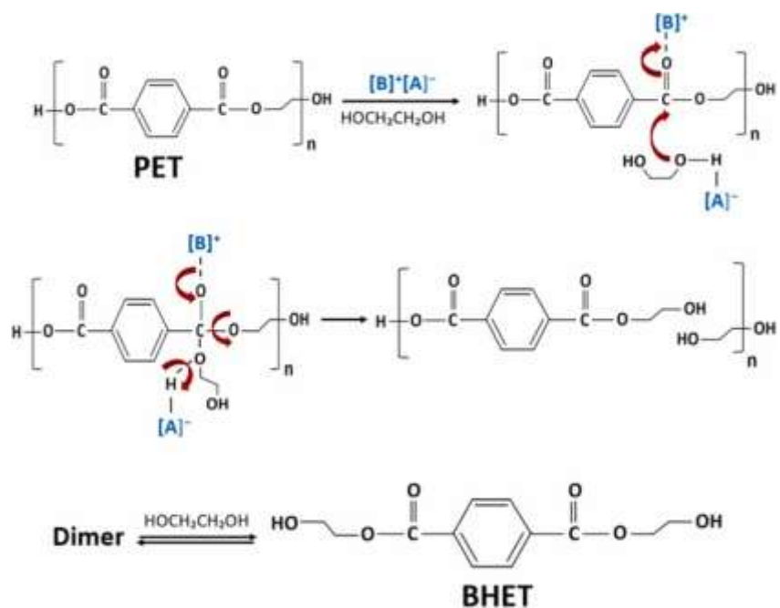
Figura 20: Mecanismo de despolimerización del PET por glicólisis con etilenglicol. Fuente: Hu y otros (2025) [34].
