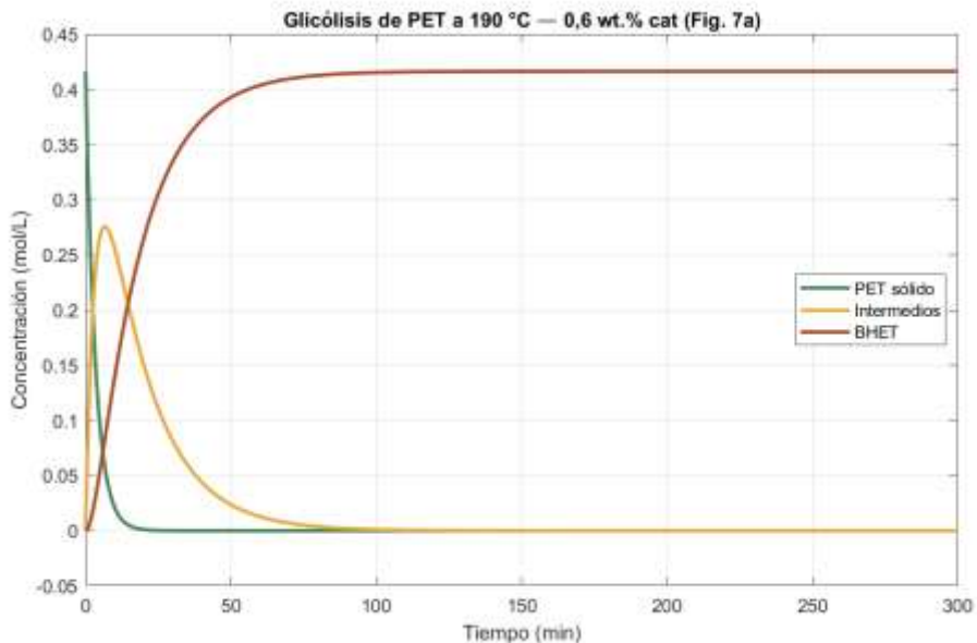
Gráfica 1: Perfil de glicólisis catalítica de PET a 190 °C con 0,6 % en peso de \text{Zn}(\text{OAc})_2 . Reproducción MATLAB del modelo de Gabrič y otros (2025) [37].
