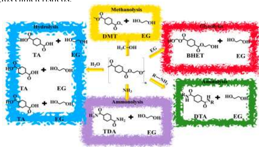
Figura 7: Procesos de reciclaje químico del PET (metanólisis, hidrólisis, glicólisis, alcoholisis y aminólisis) y sus reacciones químicas correspondientes con los productos formados. Fuente: Enache y otros (2024) [1]
